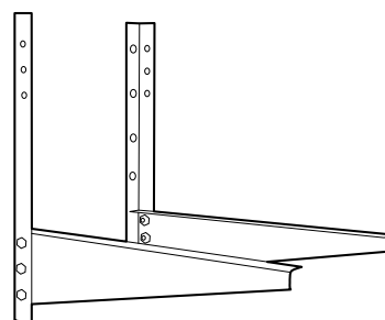
WANDHALTERUNG
